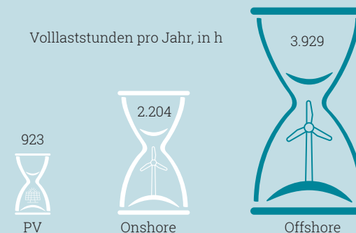
Stetige Energie: Durchschnittliche Jahresvolllaststunden aller Solar- und Windenergieanlagen in Deutschland bis 2040 Quelle: Übertragungsnetzbetreiber
